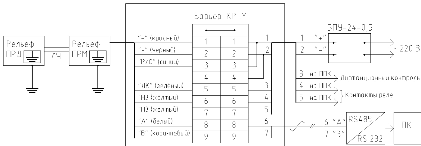
Рисунок 2.7 – Схема подключения извещателя в режиме контроля (индикатор включен).
