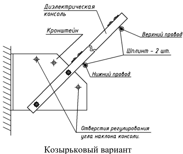
Рисунок 2.5 – Крепление проводов линейной части извещателя
