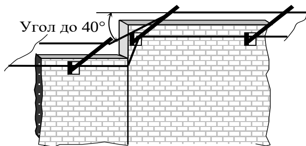
Рисунок 2.3 – Крепление КМЧ и проводов при перепадах высоты
