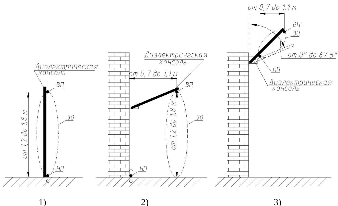
Рисунок 2.1 – Варианты размещения линейной части извещателя
