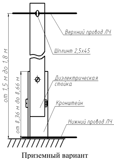
Рисунок 2.5 – Крепление проводов линейной части извещателя
