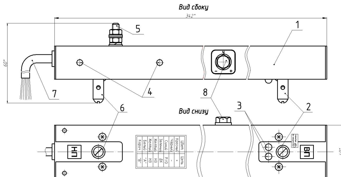
Рисунок 1.3 – Конструкция ПРМ.
