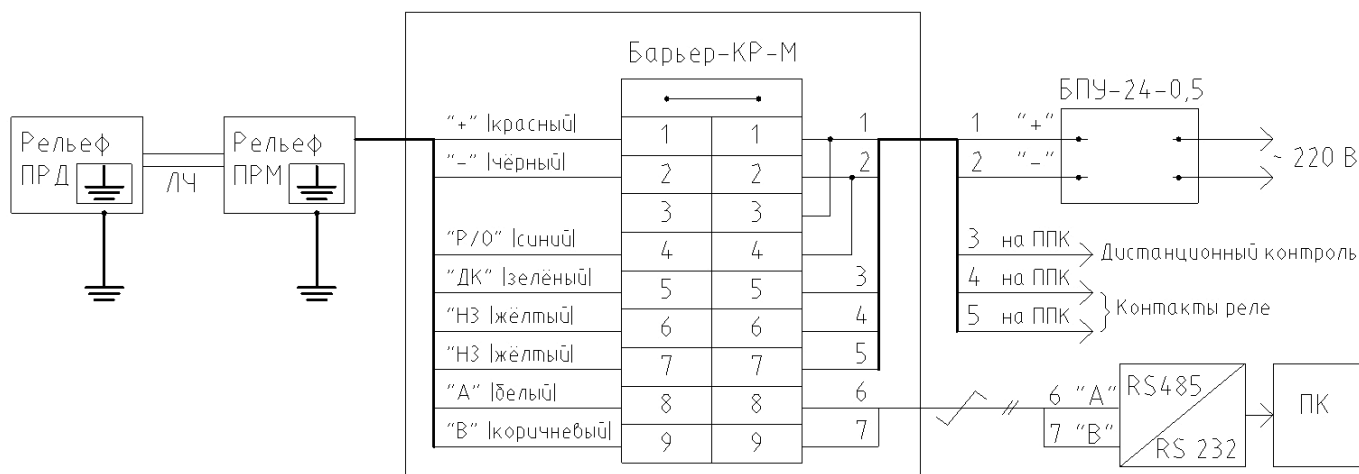
Рисунок 2.9 – Подключение извещателя к коробке распределительной в режиме настройки чувствительности (индикатор выключен).
