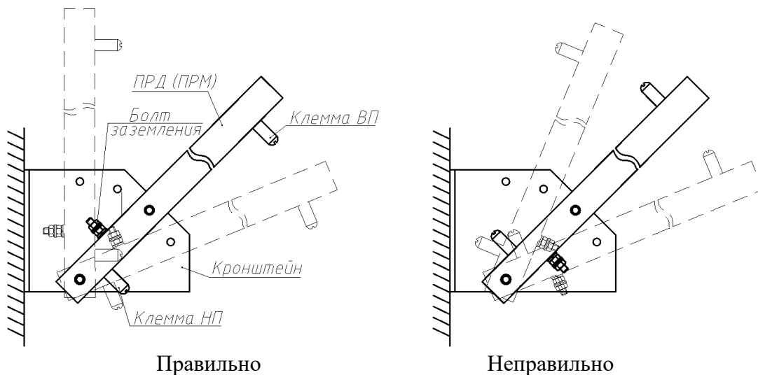
Рисунок 2.6 – Установка ПРД и ПРМ
